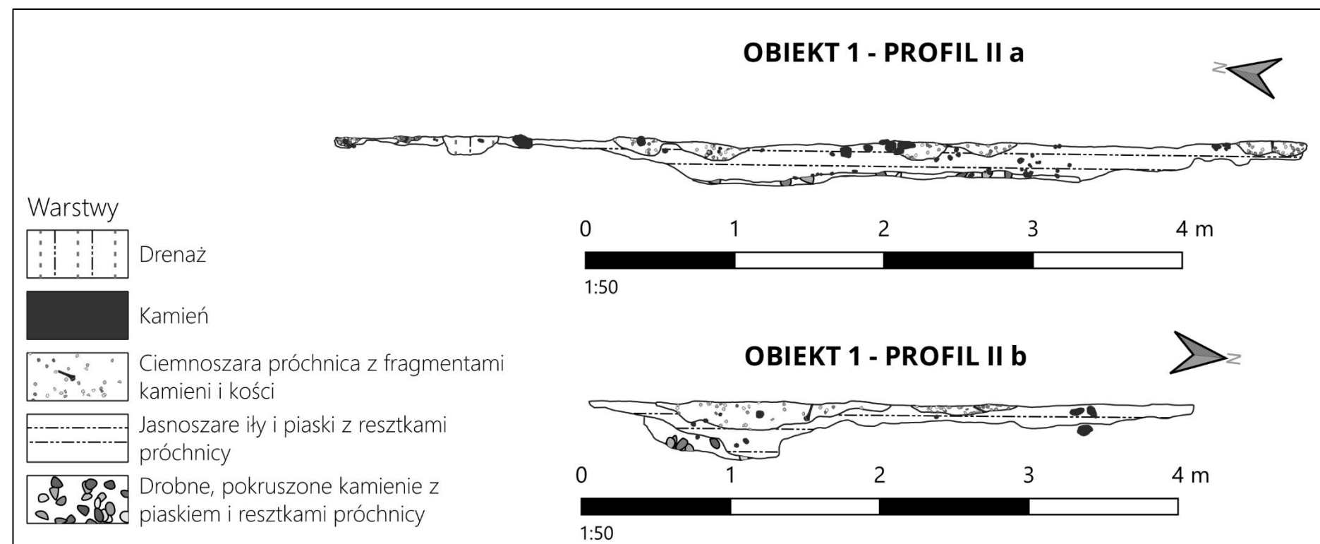
Ryc. 14/26 Profile IIa, IIb obiektu 1.
