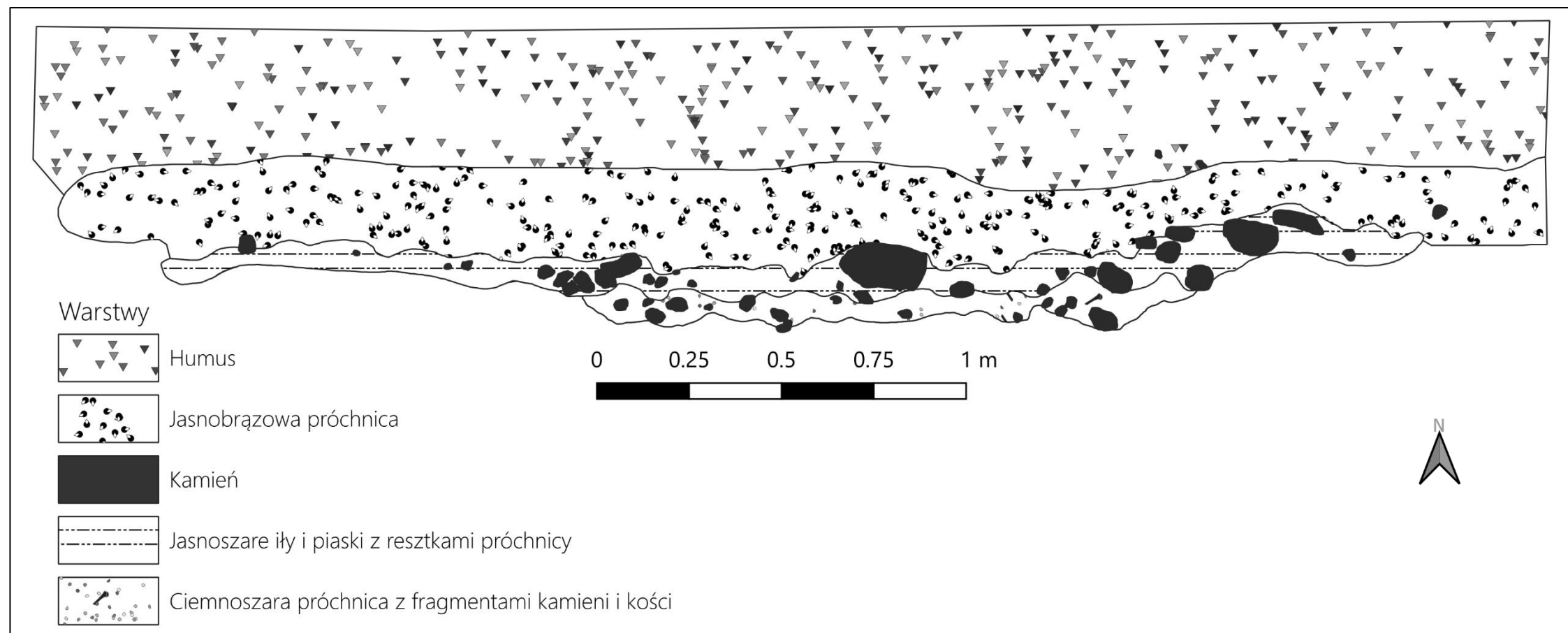
Ryc. 10/26 Profil N obiektu 1.
