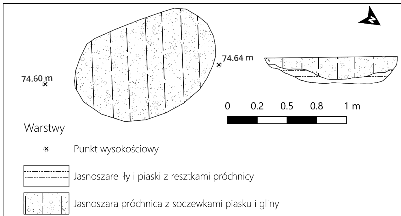
Ryc. 8/26 Rzut pionowy i przekrój poziomy obiektu 8.
