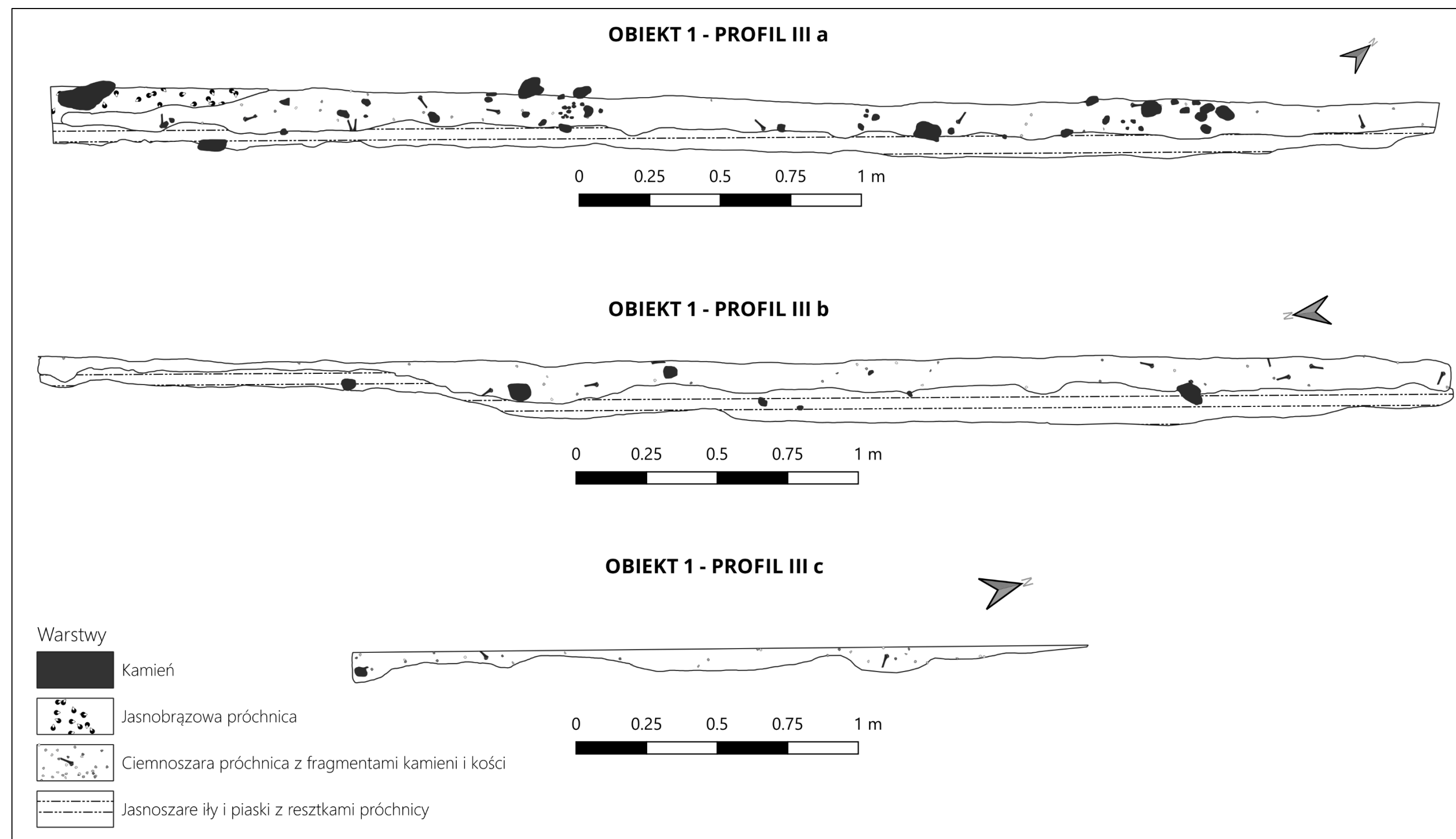
Ryc. 15/26 Profile IIIa, IIIb; IIIc obiektu 1.
