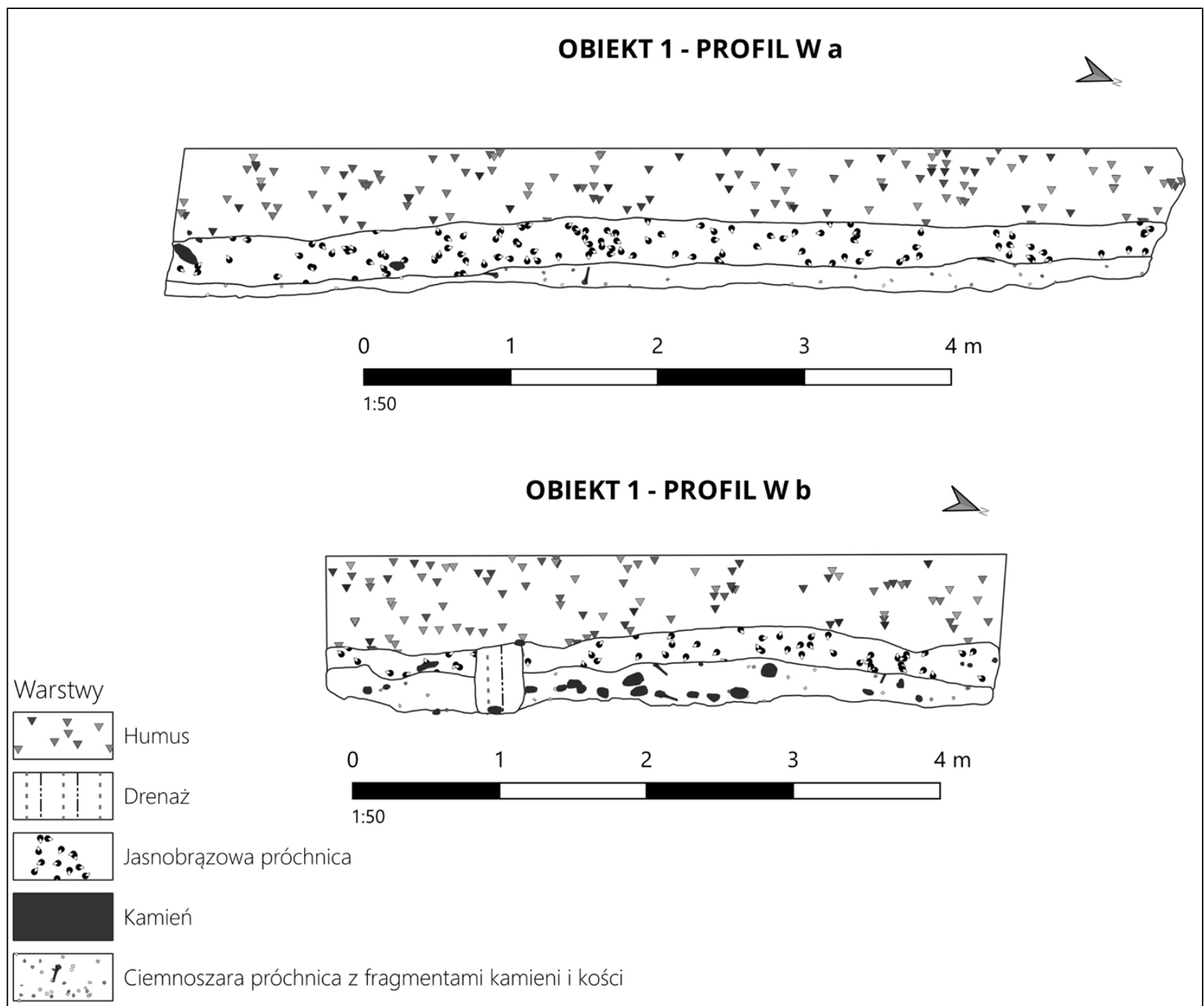
Ryc. 10/26 Profile Wa - Wb obiektu 1.
